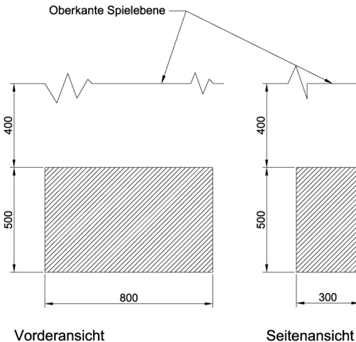
Abb. 9 Fundamentgröße Rutsche
