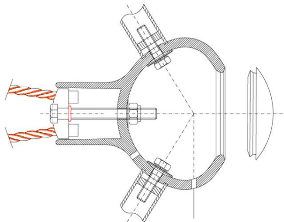
Abb. 5 Spannkugel mit Spannungspunkt
