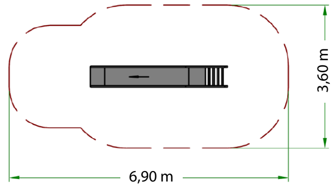
Podesthöhe 1,25-1,50 m
