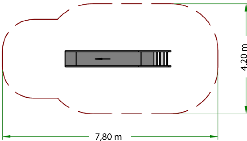
Podesthöhe 1,75-2,00 m
